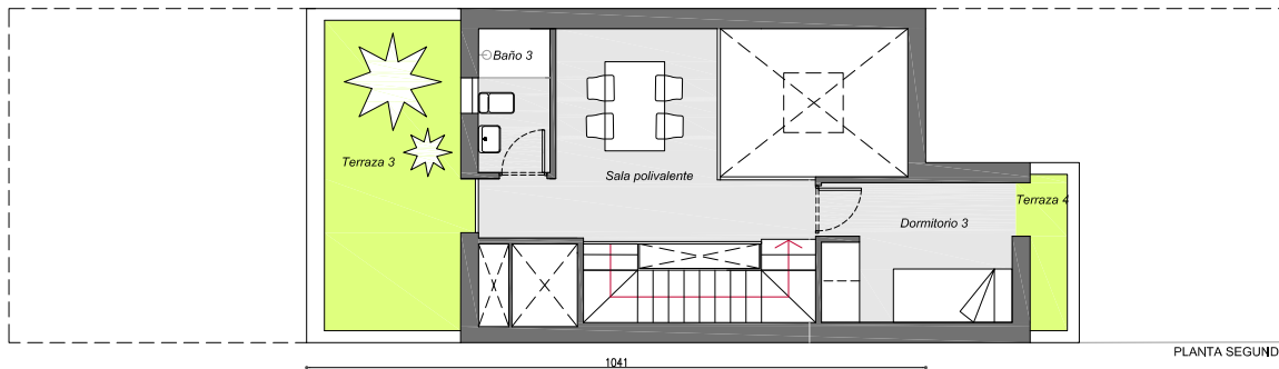
PLANTA SEGUNDA
