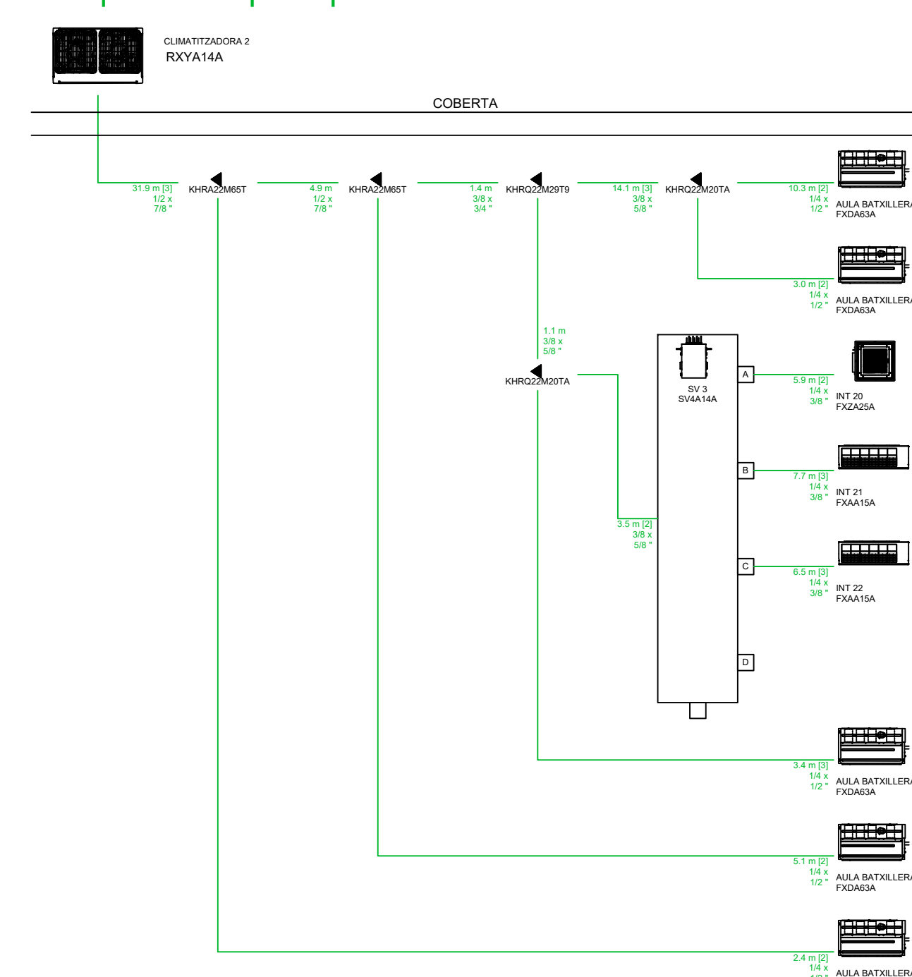
Esquema de principi - zona 2
