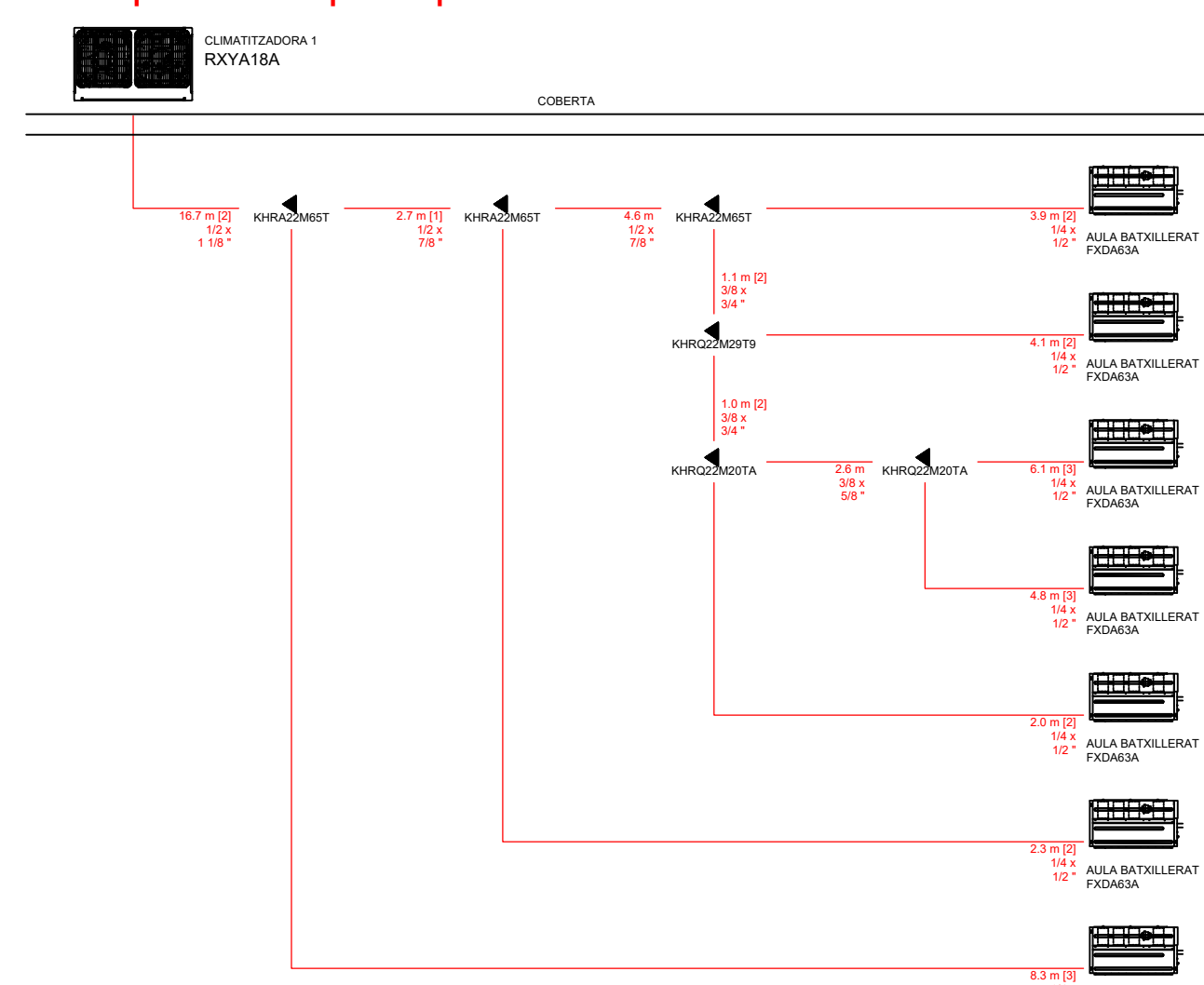
Esquema de principi - zona 1
