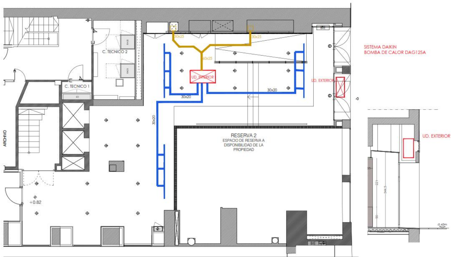
PLANO DE CLIMATIZACIÓN NUEVO ACCESO MIGUEL VILLANUEVA Miguel Villanueva , Nº 9, Logroño
