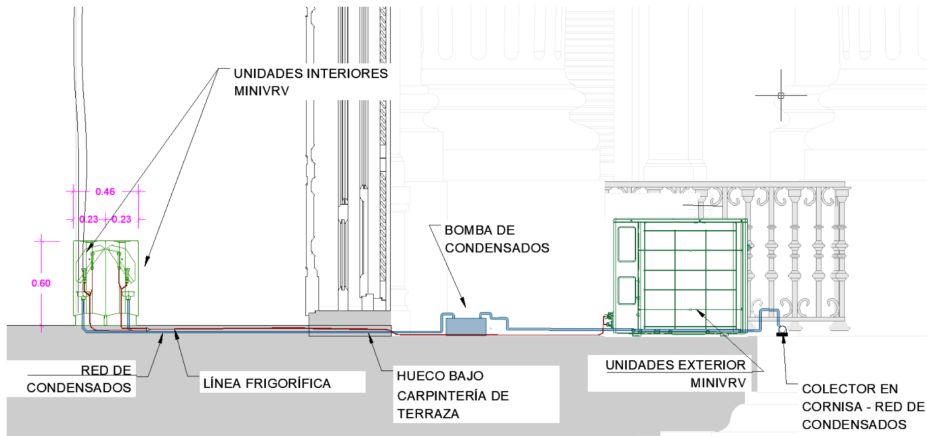
SECCIÓN DE INSTALACIÓN
