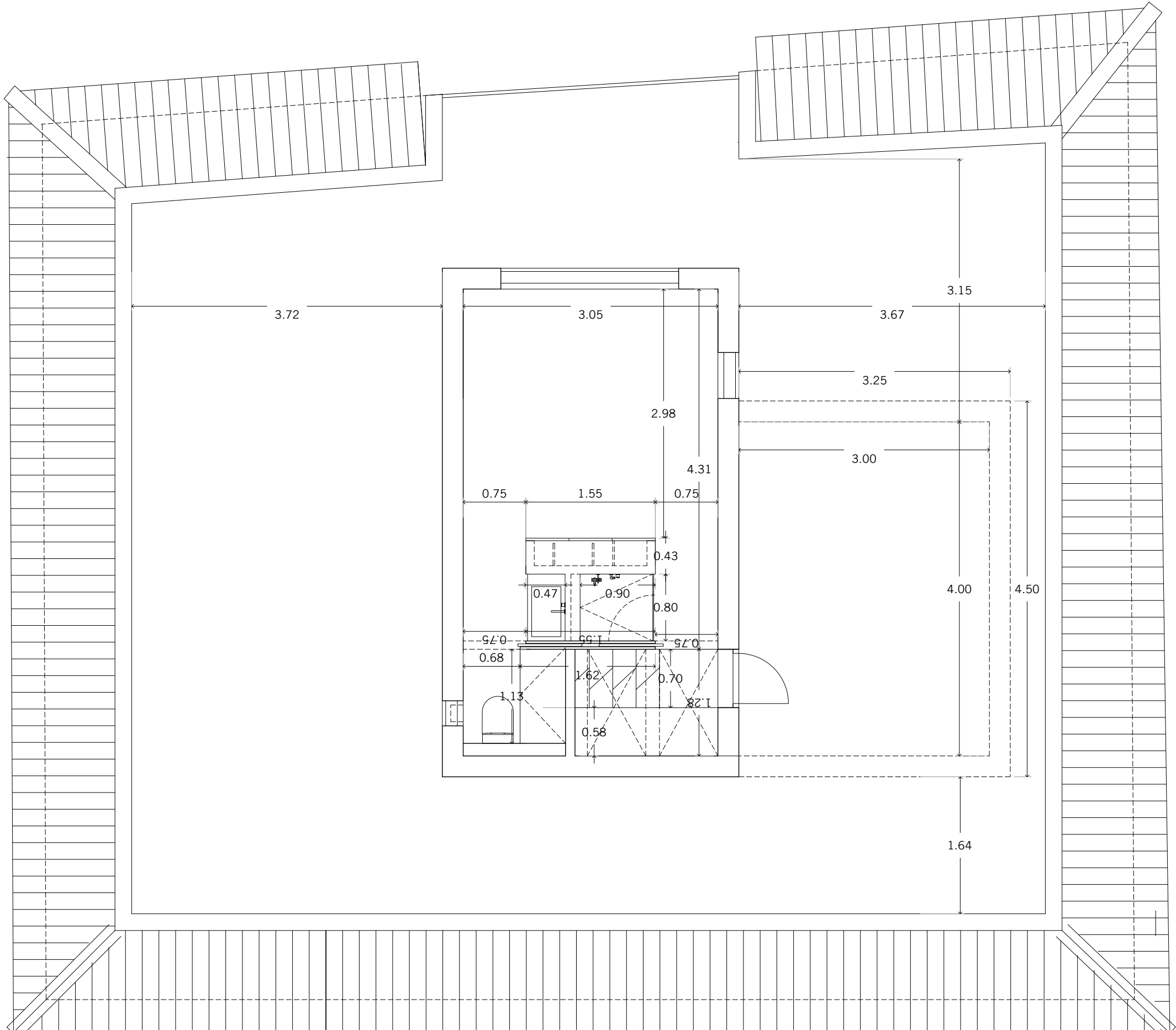
PLANTA SEGUNDA
