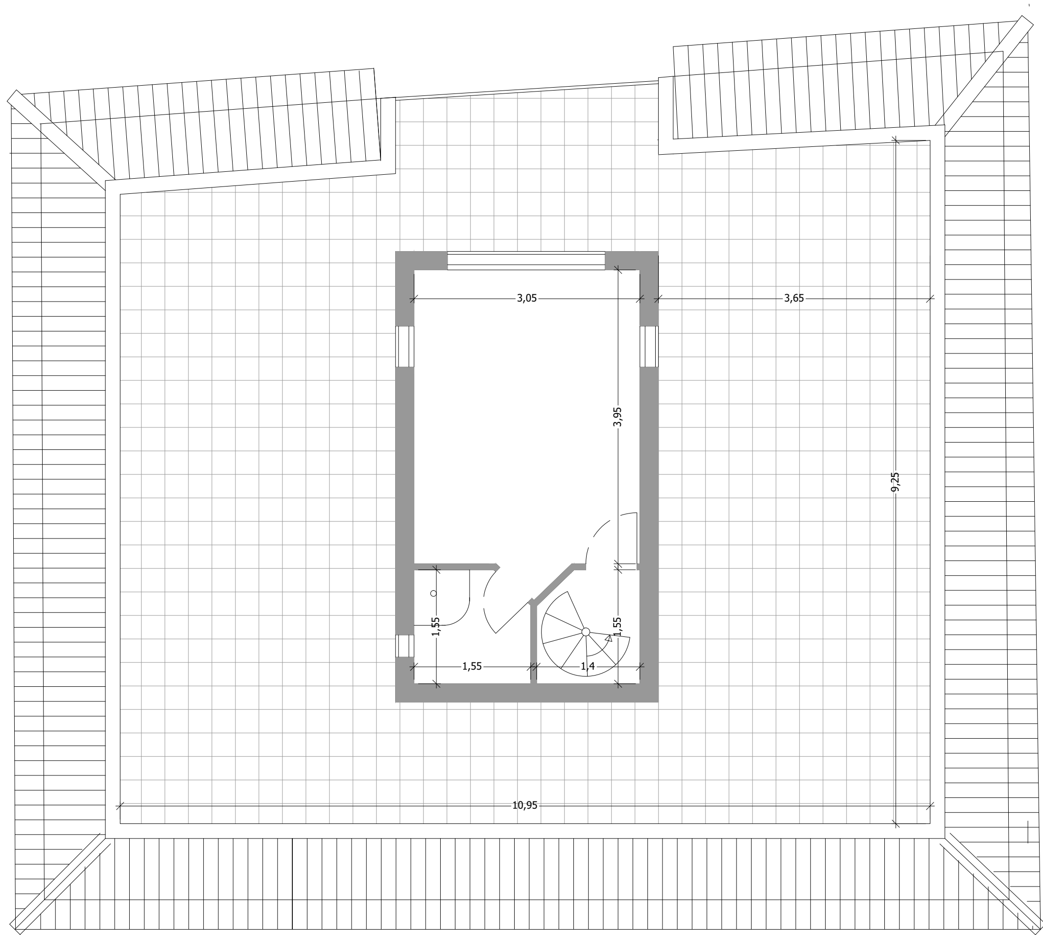
PLANTA SEGUNDA
