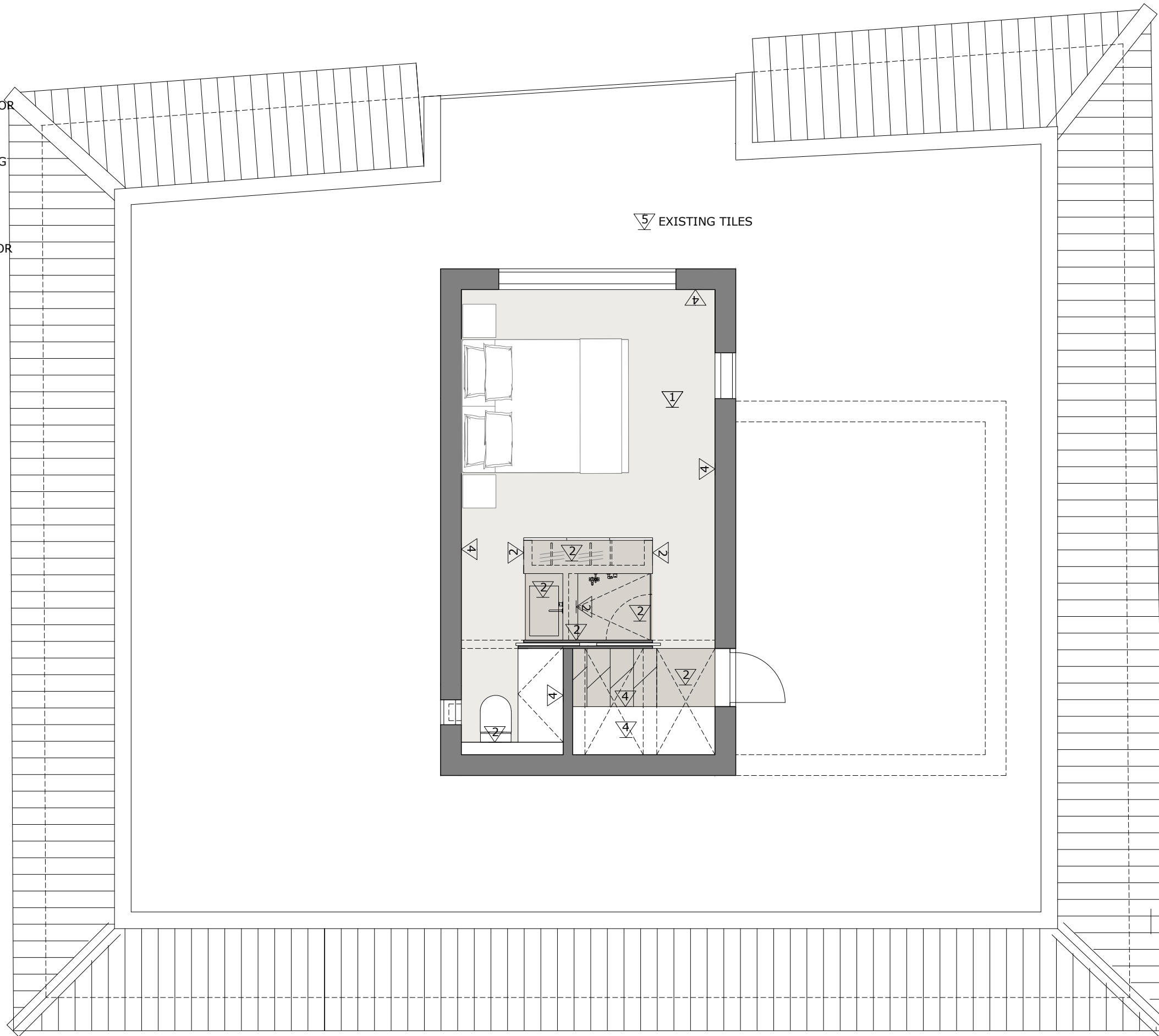
PLANTA SEGUNDA
