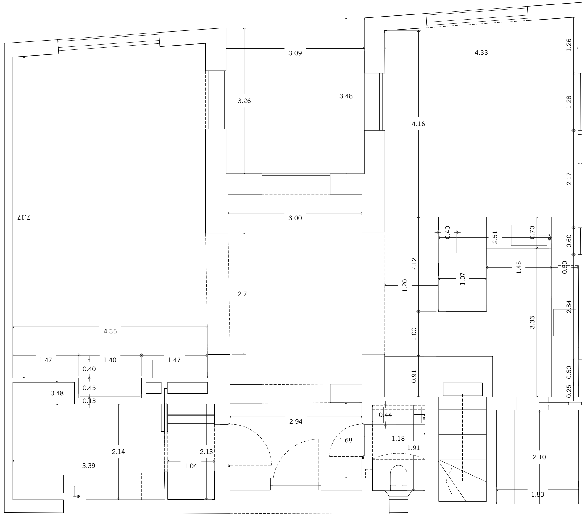
PLANTA BAJA
