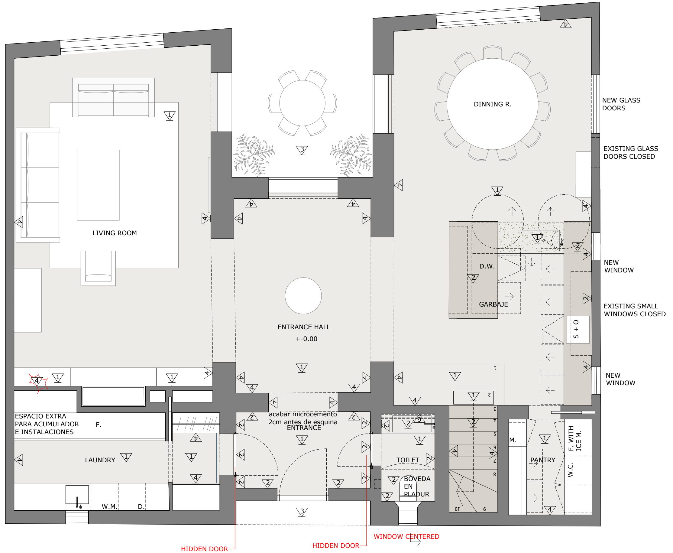
PLANTA BAJA
