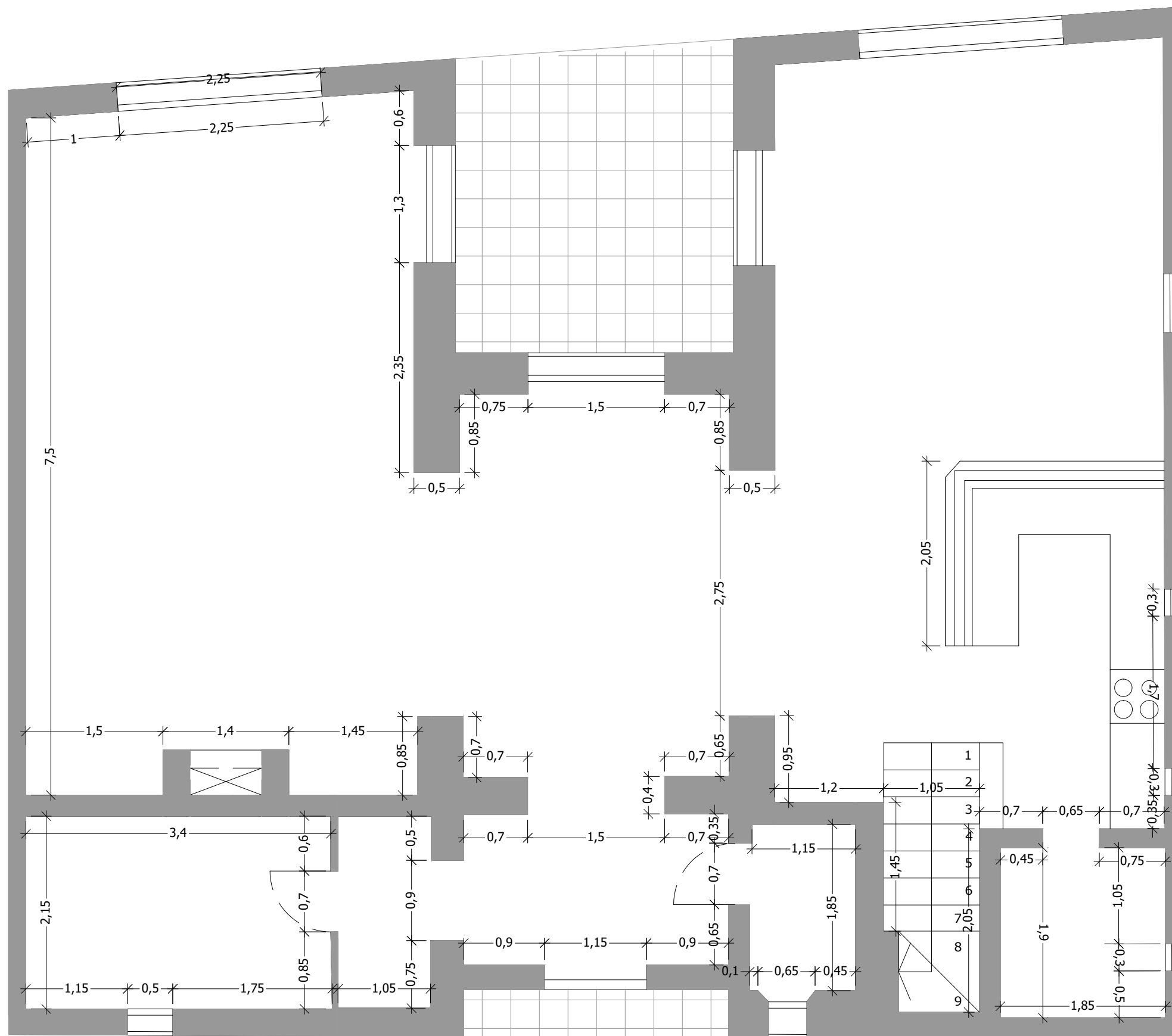
PLANTA BAJA
